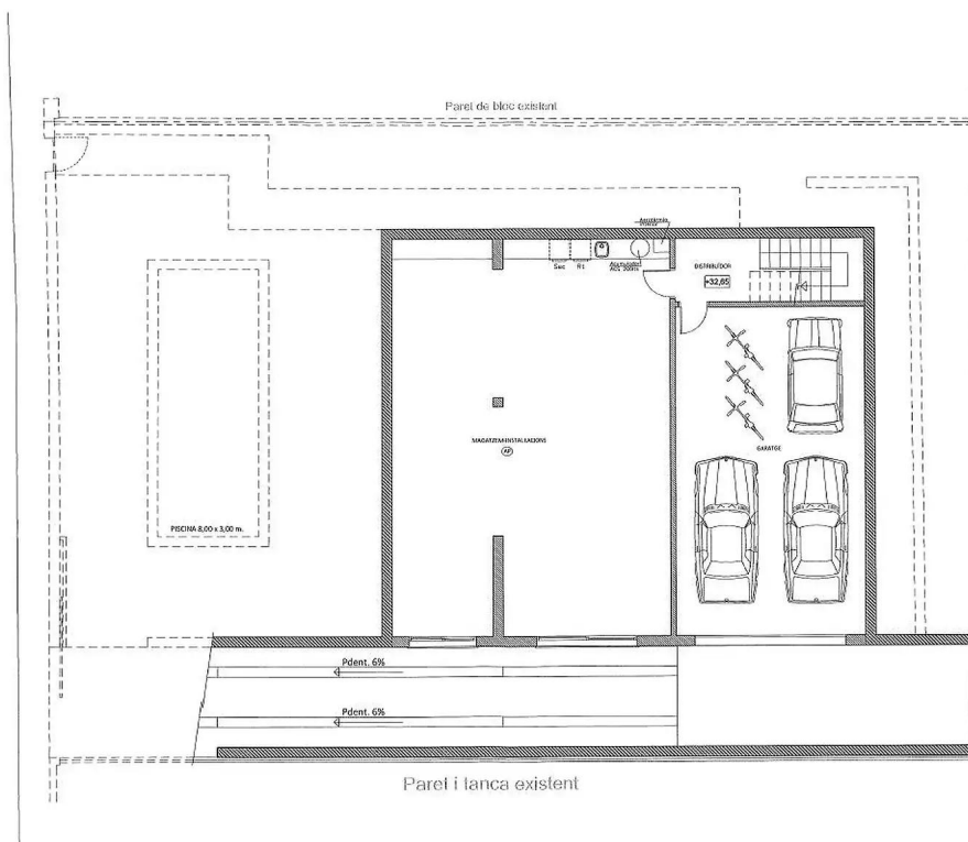
PLANTA SOTERRANI E = 1/100
