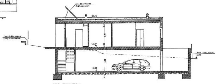
SECCIÓ TRANSVERSAL E = 1/100
